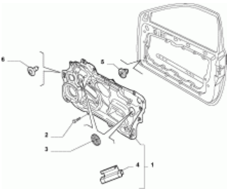
70129/00 - SIDE FRONT DOORS (Var.:2/Rev.:0)
